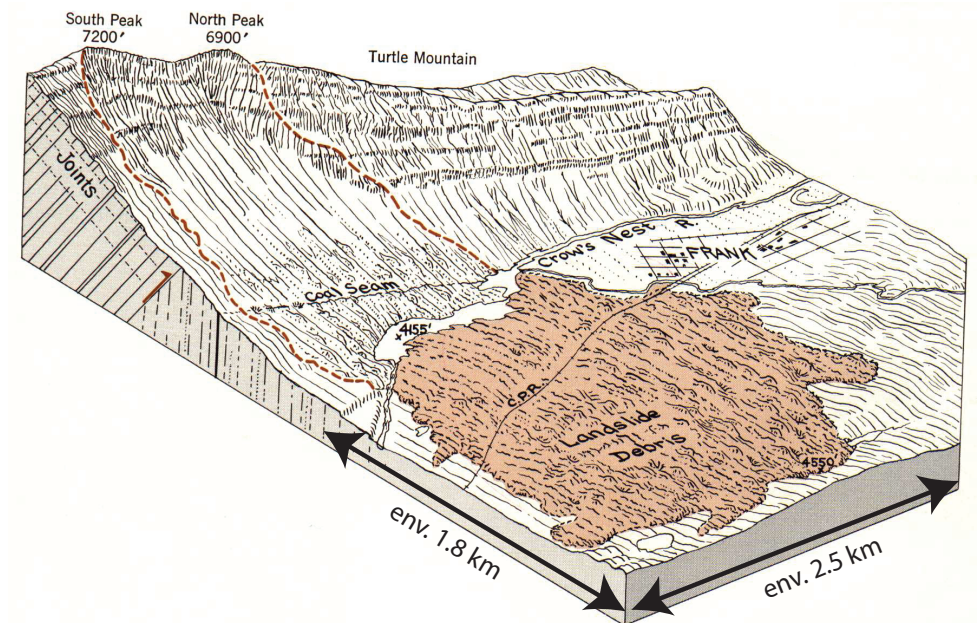
Figure 11 - Bloc-diagramme du glissement rocheux de Frank en 1903 (Alberta, Rocheuses canadiennes). Avec, à l'arrière de la masse accumulée, une zone déprimée occupée par un lac. Les altitudes sont en pieds. Image tirée de Strahler (1969). Voir aussi https://en.wikipedia.org/wiki/Frank_Slide .
