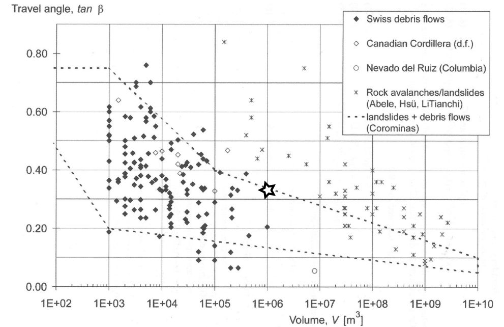
Figure 10 - Diagramme H/L - volume. Étoile = cas du Courset. X = glissements et « rock avalanches ». Graphique de base tiré de Rickenmann (2005).
