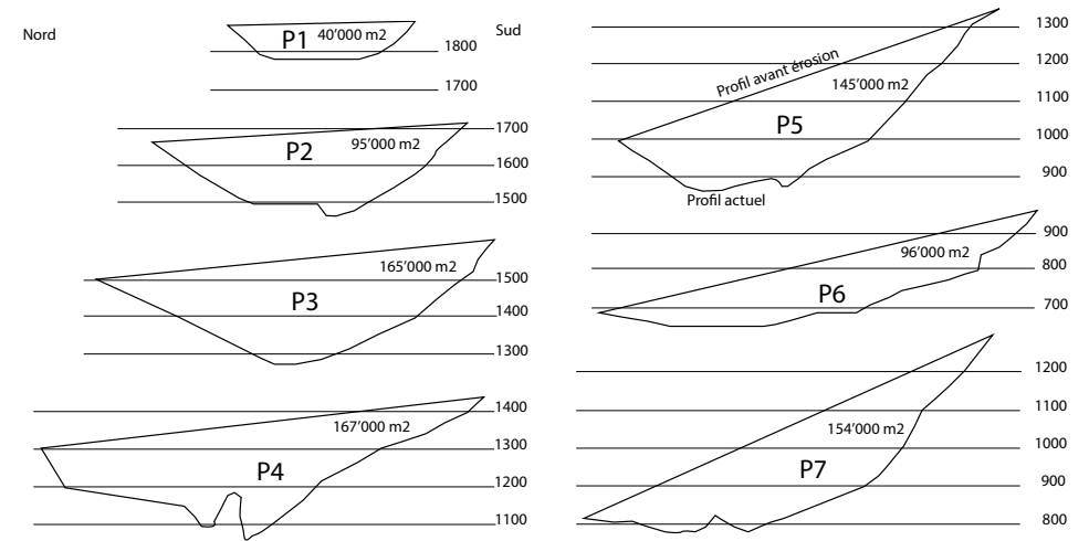
Figure 7. b) Profils en travers P1 à P7 et calcul des volumes du dièdre selon V_{tot} = V1 + V2 + V3 + V4 + V5 + V6 + V7 = 0.213 \text{ km}^3 (les superficies des profils sont pondérées par l'espace entre les profils).
