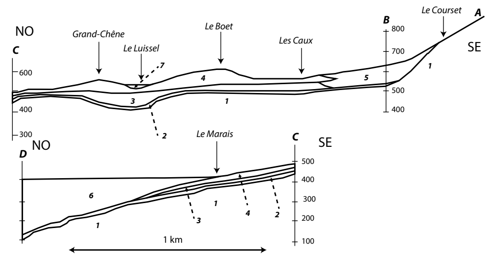
Figure 8. Profil sud-est / nord-ouest (A/D). Partant du pied du dièdre d'érosion du Courset, traversant les collines et se terminant au Marais de Bex; voir sa situation sur la figure 1. 1) substratum rocheux. 2) moraine de fond. 3) premier éboulement. 4) second éboulement. 5) sédiments de cône de déjection. 6) alluvions du Rhône. 7) sédiments palustres.
